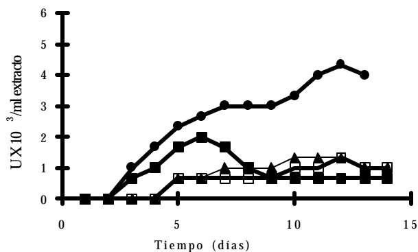
Fig. 1. Actividad feruloil, cafeil y p -cumaroil esterasa de A. awamori . ácido ferúlico (●), ácido caféico del ácido clorogénico (■), ácido caféico del metil cafeato (□), ácido p -cumárico (♦)
