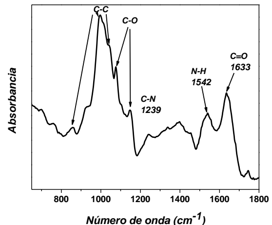
Fig. 1. Espectro característico de infrarrojo de un grano de frijol.
